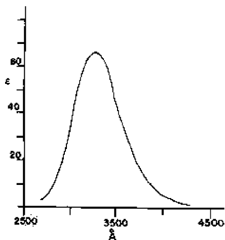
Рис. V-16. Коэффициенты поглощения \text{Cl}_2 в области 2500 – 4500 Å [393]. Коэффициент \epsilon выражен в л/ (моль · см), основание 10, температура комнатная. [Copyright 1933 by the American Institute of Physics.]
