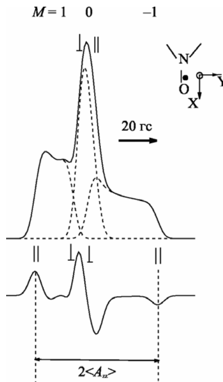
Рис. 2. Форма спектра ЭПР нитроксильного радикала в отсутствие движений (Расчет по формуле (3)). Внизу приводится спектр в виде первой производной по полю. Пунктиром показаны отдельные сверхтонкие компоненты. Для каждой из них указаны примерные положения параллельной и перпендикулярной ориентаций. На врезке показана молекулярная система координат)
